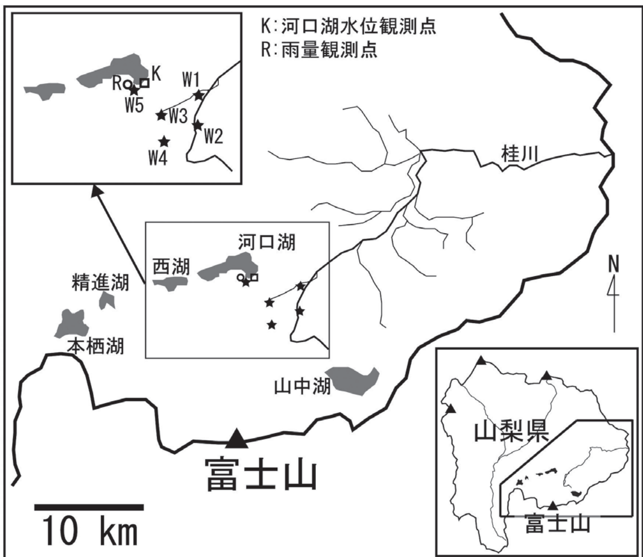
図1 河口湖南東部の井戸の位置（国土交通省河川局 4) の水系図，尾形ら 5) をもとに作成）
