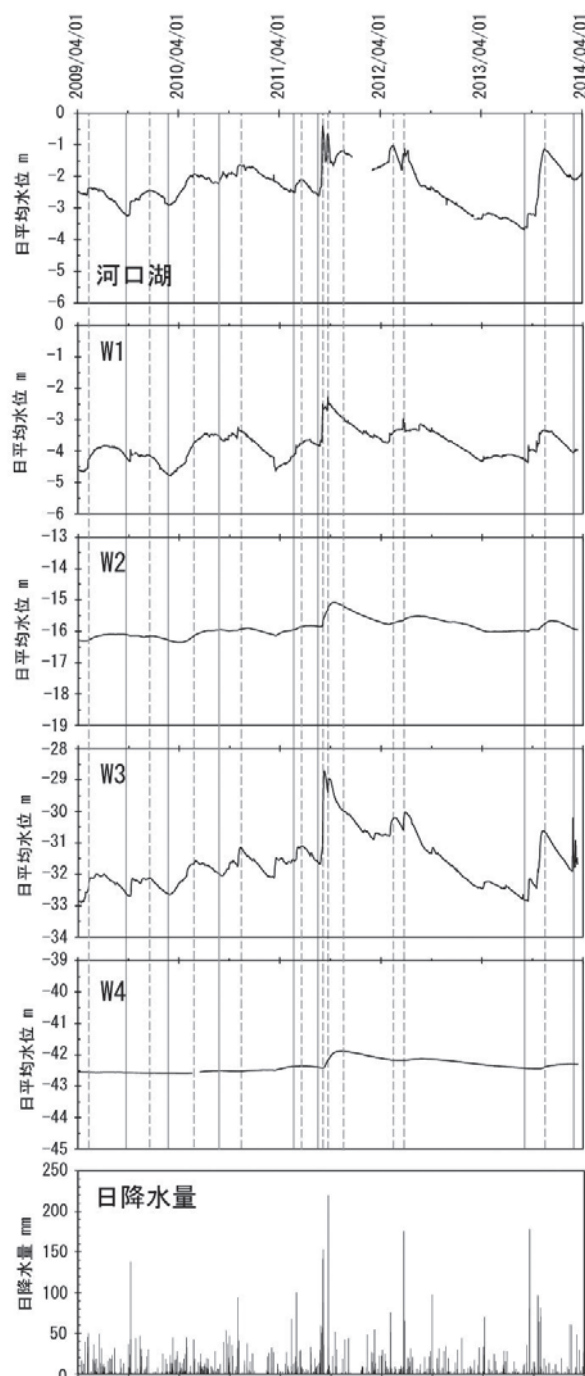
図2 河口湖の水位, 降水量と河口湖南東部W1からW4の地下水位の経時変化 (河口湖の水位は山梨県 6) をもとに作成, 日降水量は気象庁 7) をもとに作成)。実線は河口湖の水位低下のピーク。点線は河口湖の水位上昇のピーク。
