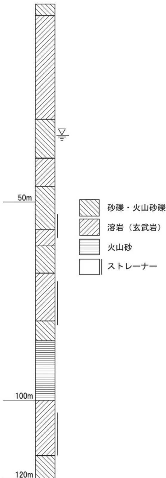
図3 河口湖南東部W5の地質柱状図(尾形ら 5) )
