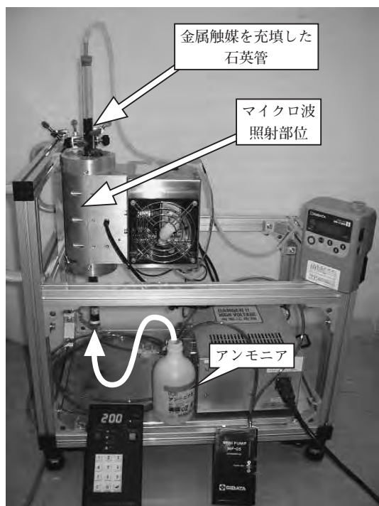
写真-9 マイクロ波分解装置
