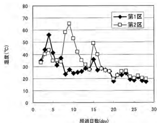
図-1 発酵温度の変化
