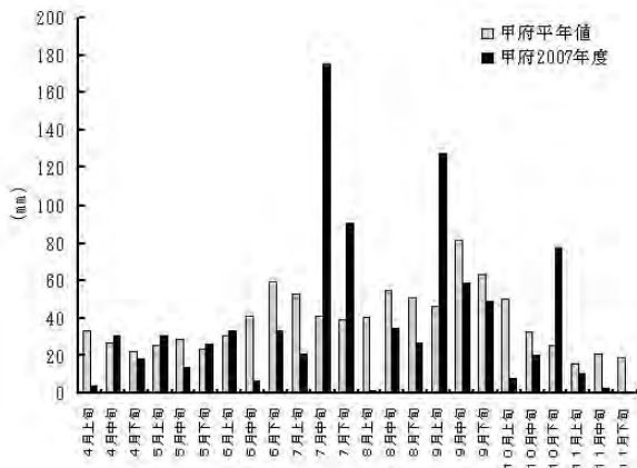
図2 甲府における2007年度の降水量と1971～2000年の の平年降水量
